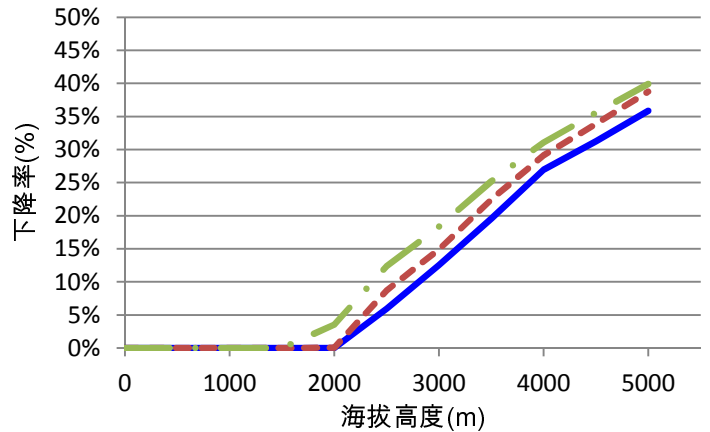
额定功率
